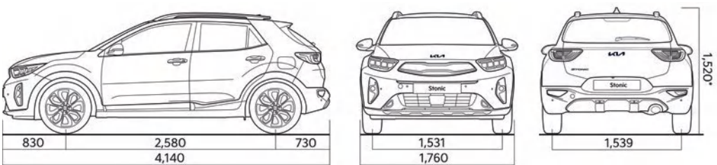
Dimensões (mm) *Com barras de tejadilho
